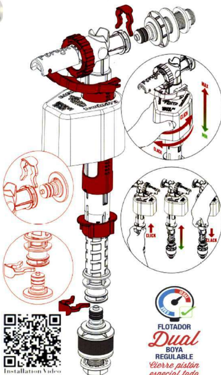
ALIMENTACIÓN UNIVERSAL POSICIÓN INFERIOR VÁLIDO PARA CISTERNAS CON ENTRADA DE AGUA INFERIOR
